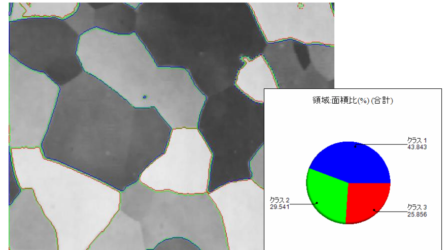
合金の各種金属の組成含有率
