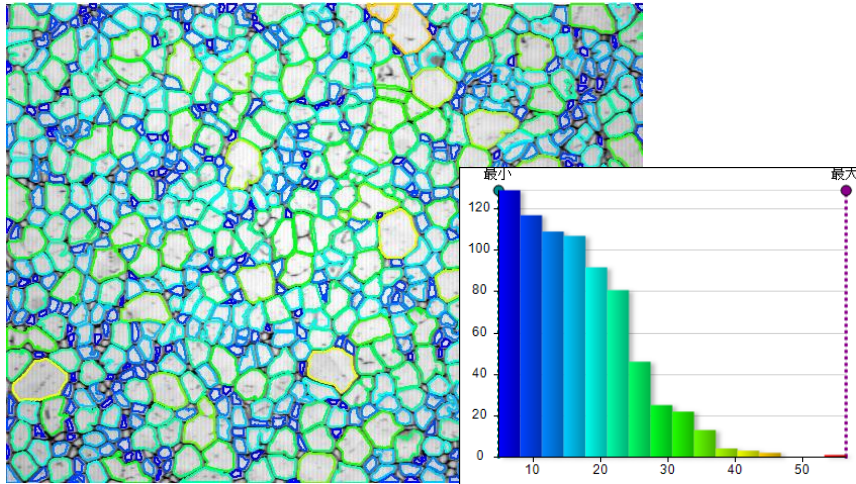
金属グレインの長径・短径測定
